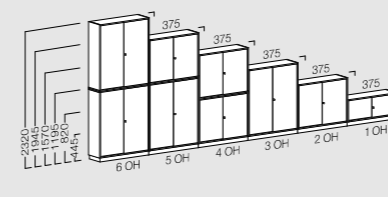
Schiebetürenschränke SHU/SHA
