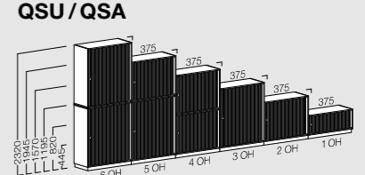
Querrollladenschränke QSU/QSA
