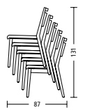
6510 / 6511 Max. 5 Stühle mit Stapel- wagen 6491-000.
