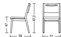
6510 ungepolstert / 7,5 kg gepolstert 8,0 kg
