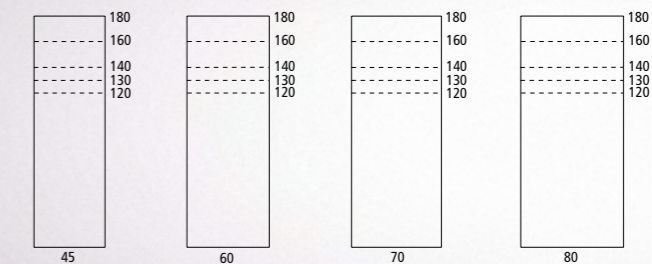
Klapptische mit T-Fußgestell
