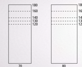
Klapptische mit 4-Fußgestell, Fußquerschnitt quadratisch
