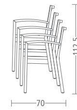
Stapelbarkeit Modelle 6710 und 6711
