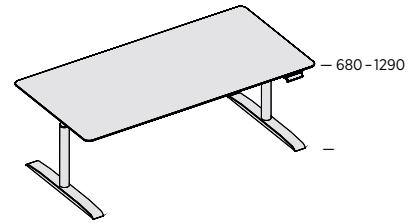
Desk with electric height adjustment | Schreibtisch mit elektromotorischer Höhenverstellung
