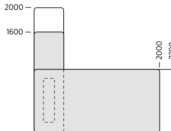
Rectangular for integration with a fixed sideboard | Rechteckig zur Verbindung mit stationärem Sideboard
