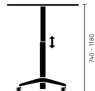
Lifftisch mit Fußkreuz auf Rollen
